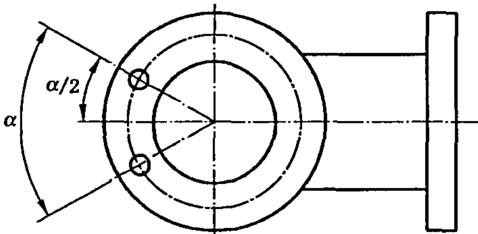
图 1 螺栓孔位置
