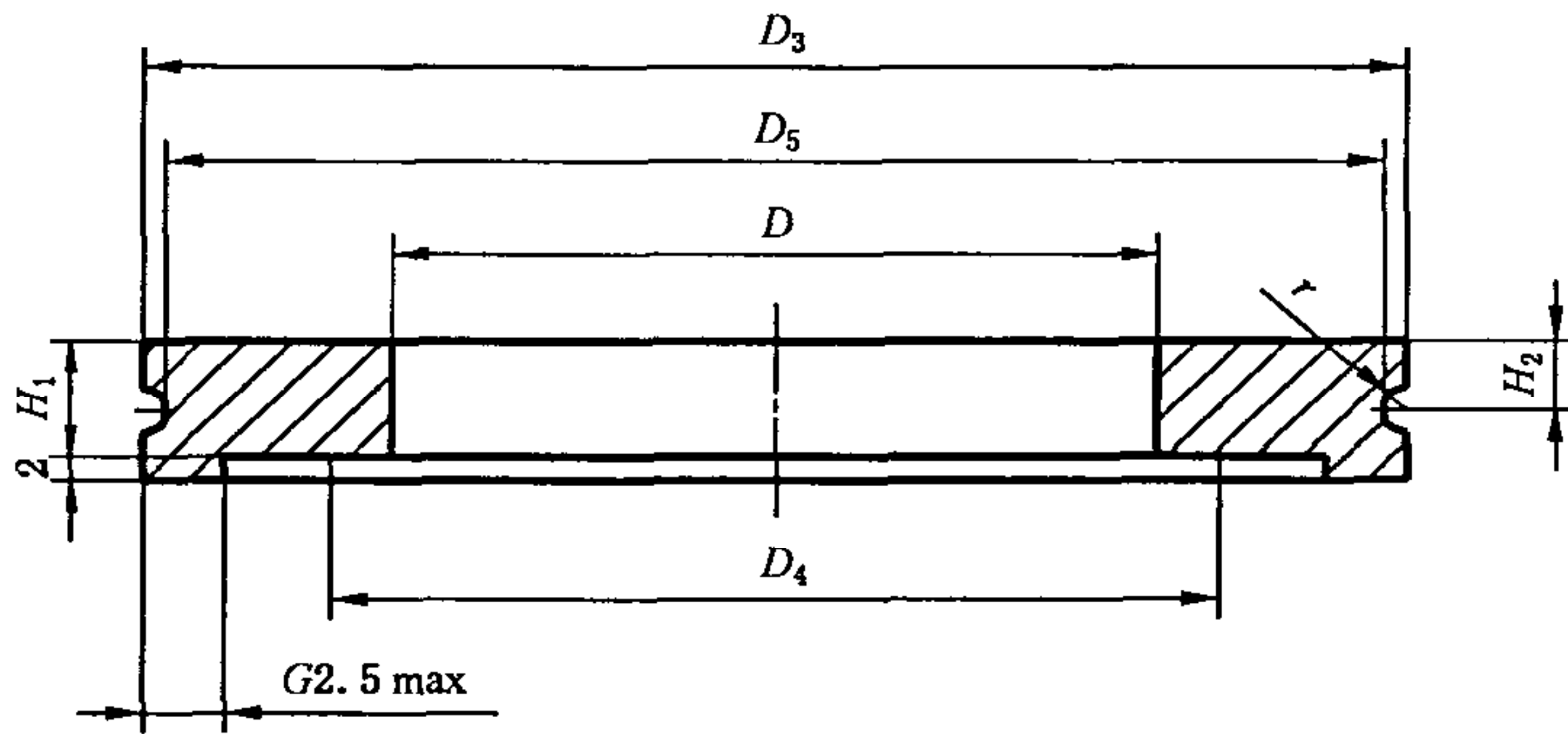
图 3 卡钳法兰
