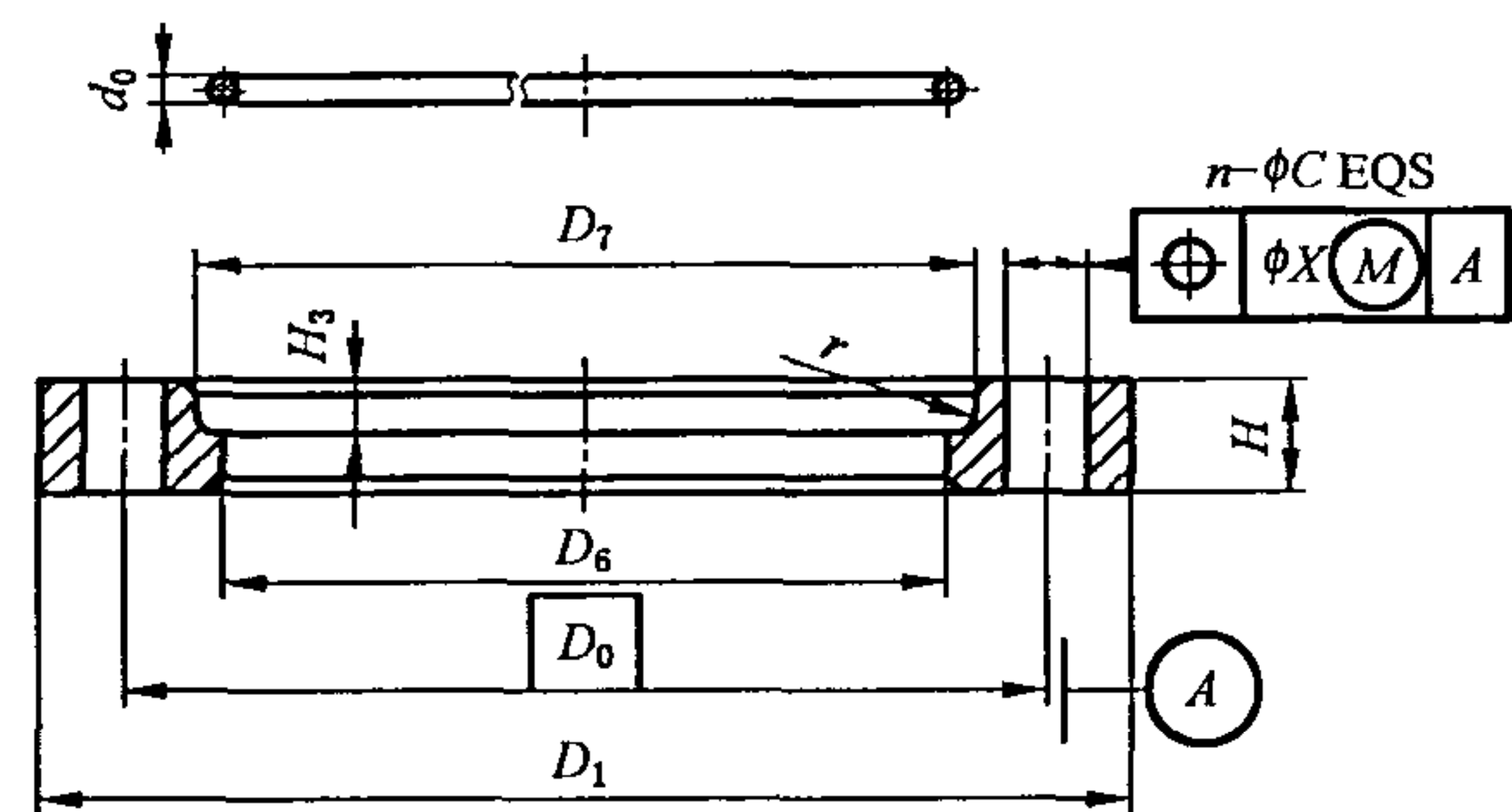
图 4 活套法兰 表 3 活套法兰尺寸
