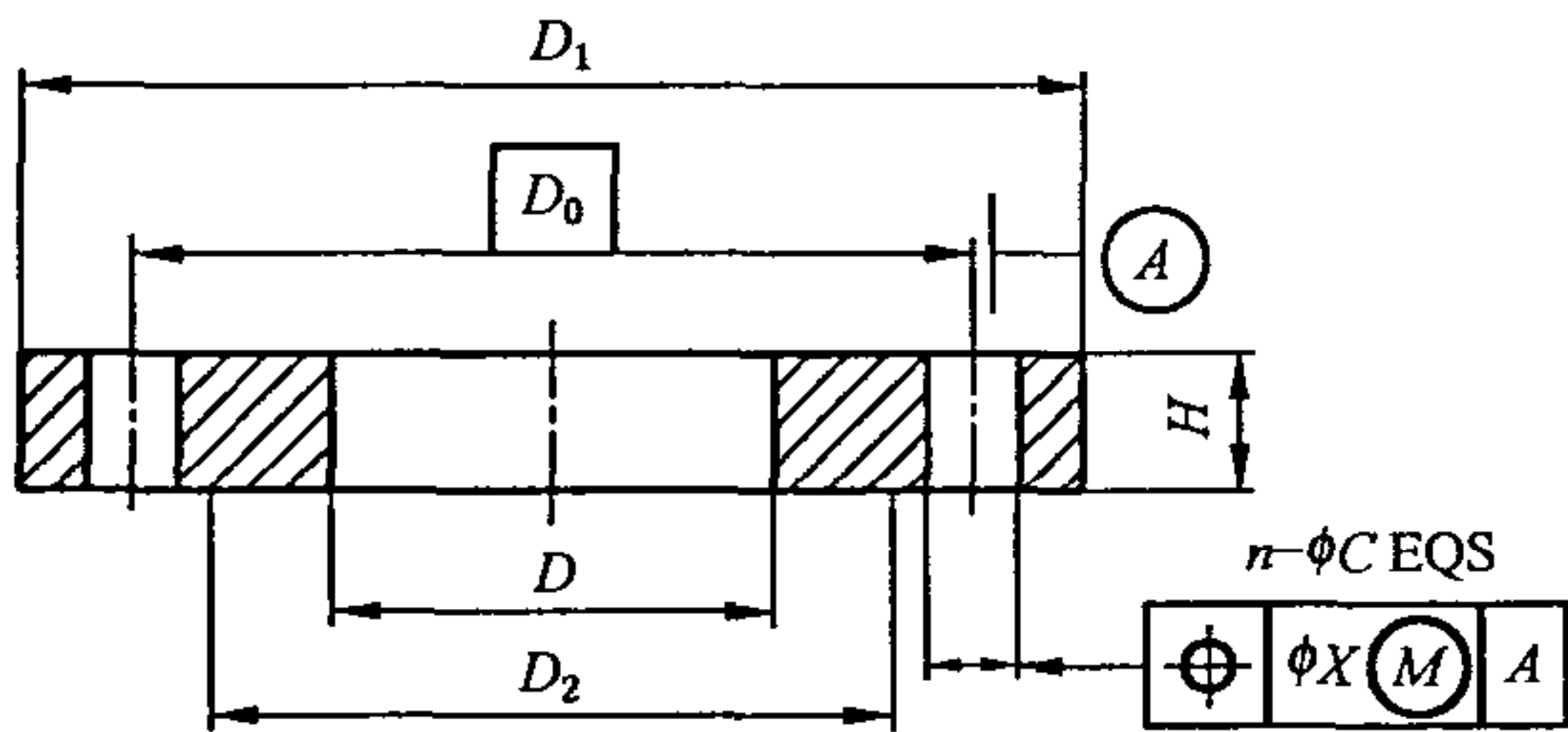
图 2 固定法兰
